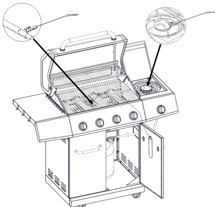
Quemador Principal
