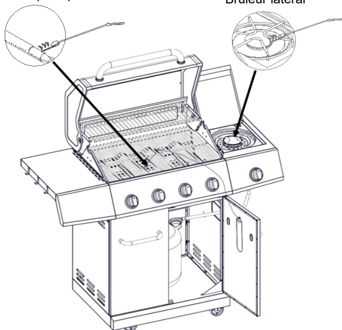
Brûleur principal
