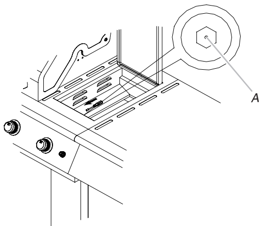
A. Gicleur
