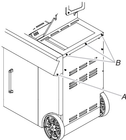
A. Tornillo del panel de control del asador B. Tornillos del estante lateral del asador
