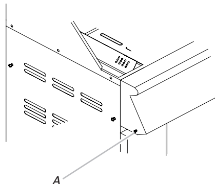
A. Vis du tableau de commande du gril
