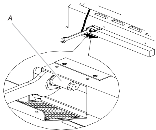
A. Tuerca del orificio
