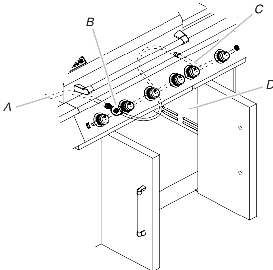
A. Tuyau à gaz en PVC de 10 pi. (3 m) B. Ensemble détendeur pour gaz naturel/tuyau C. Tubulure de distribution D. Panneau de droite
