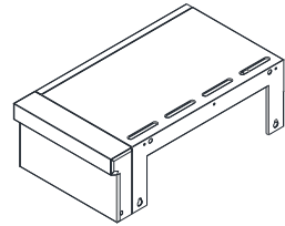
B. Étagère latérale, gauche—1 unité
