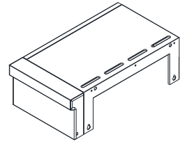
B. Estante lateral izquierdo—1 pieza
