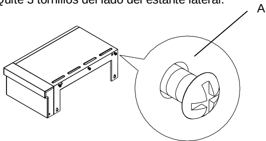
A. Tornillos del estante lateral
