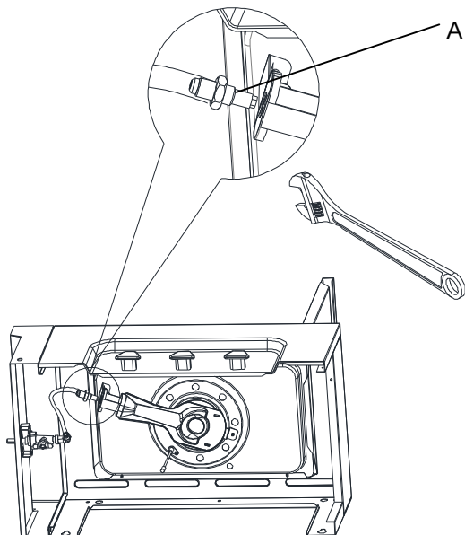
A. Side burner flex end
