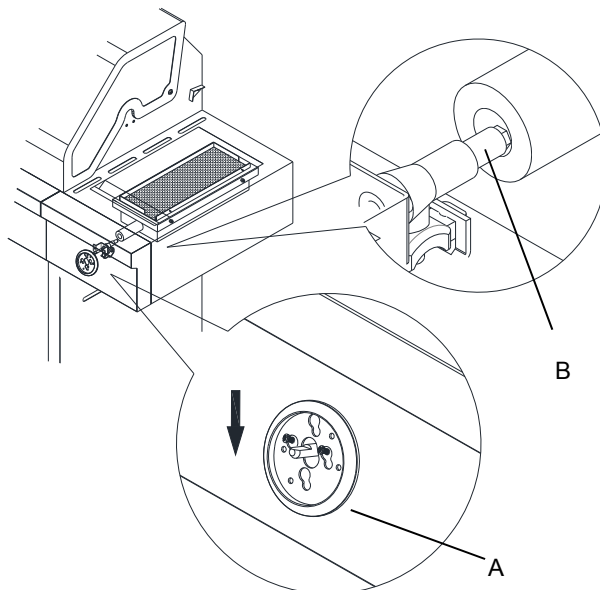
A. Collerette B. Tige de la valve
