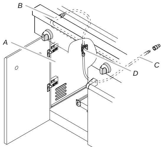
A. Panel lateral izquierdo B. Distribuidor C. Manguera de gas en PVC de 10 pies (3,0 m) D. Ensamblaje de regulador de presión/ manguera de gas natural
