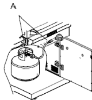
A. Ensemble détendeur/tuyau
