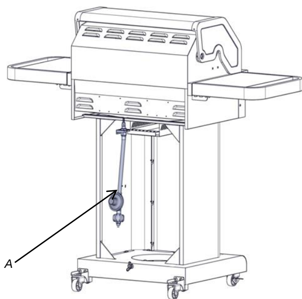
A. Ensemble détendeur/tuyau
