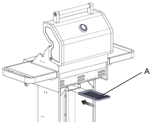
A. Recipiente para grasa
