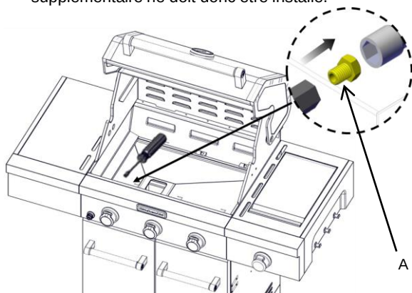
A. Gicleur de brûleur principal
