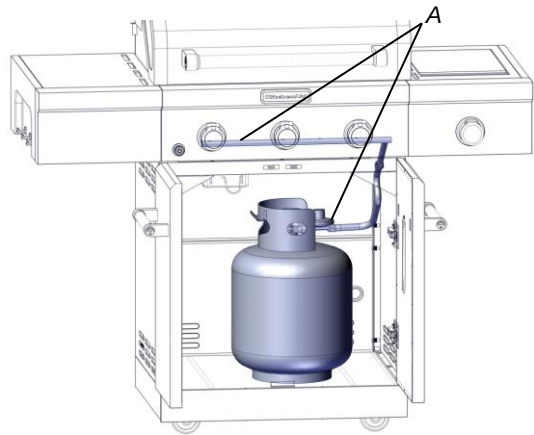
A. Ensemble détendeur/tuyau
