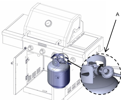
A. Ensemble détendeur/tuyau
