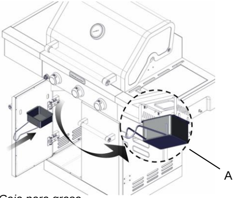
A. Caja para grasa
