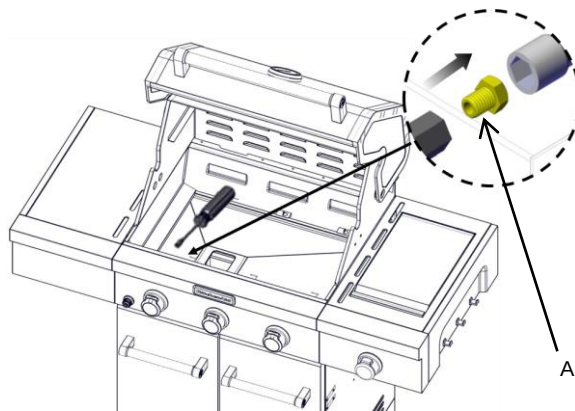
A. Orificio del quemador principal
