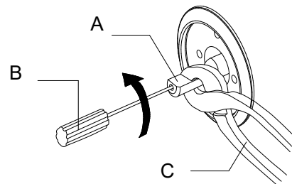
A. Valve stem
