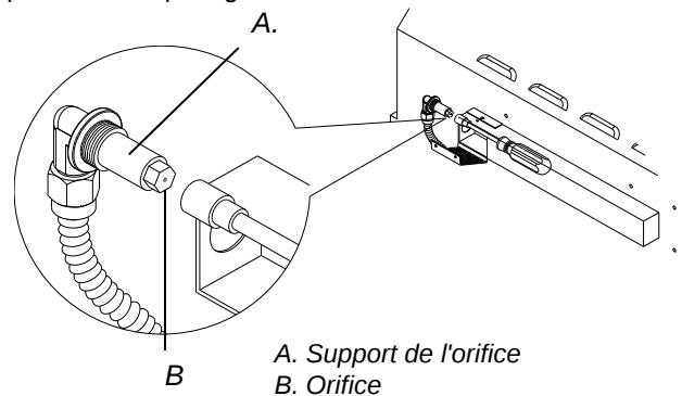
B. Orifice
