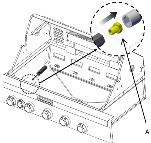
A. Main burner orifice
