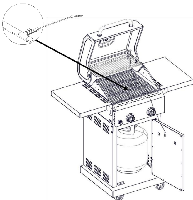
Brûleur principal
