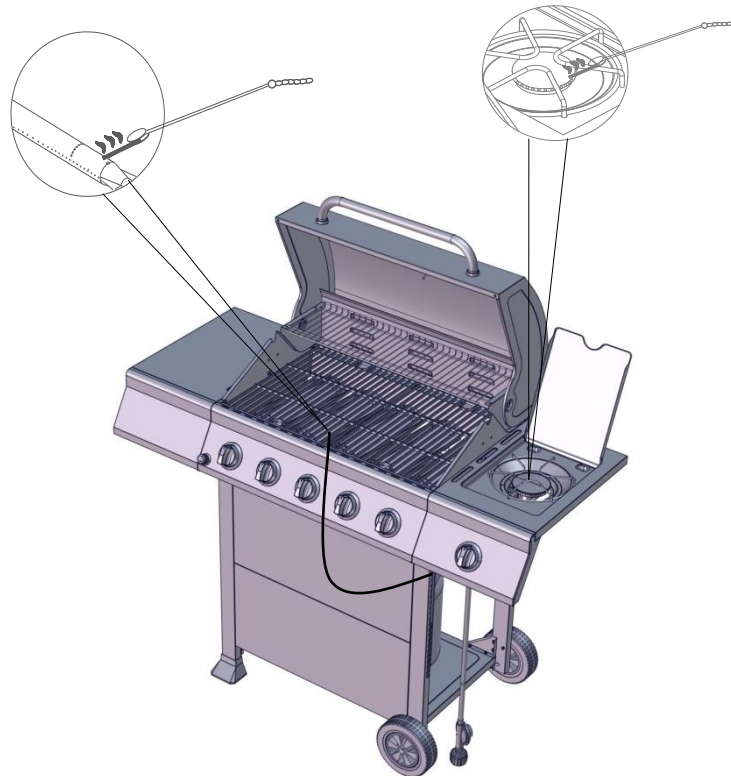
brûleur principal
