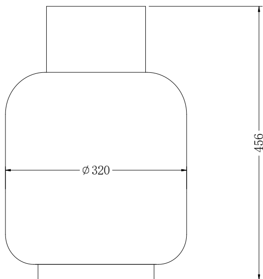
Réservoir de propane : hauteur = 456mm , diamètre = 320mm
