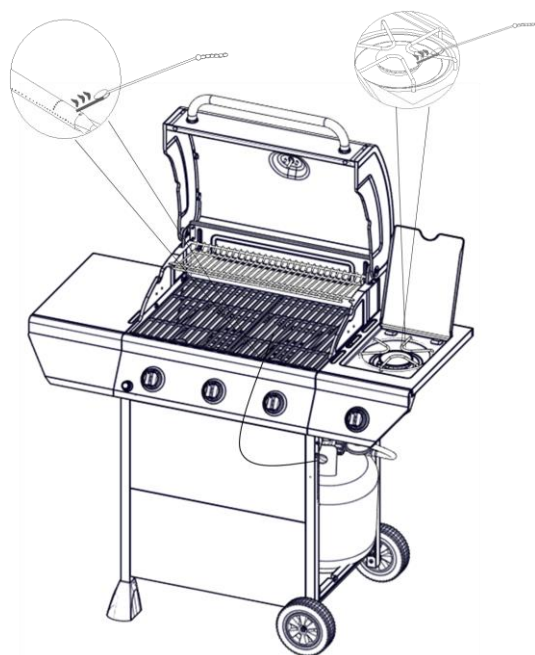
Brûleur Principal
