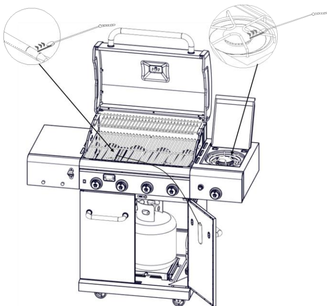
Brûleur principal
